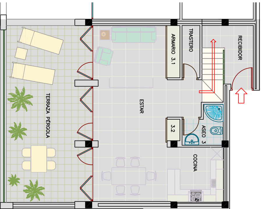
PLANTA INFERIOR
