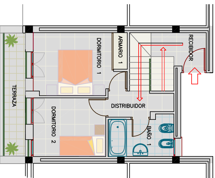
PLANTA SUPERIOR
